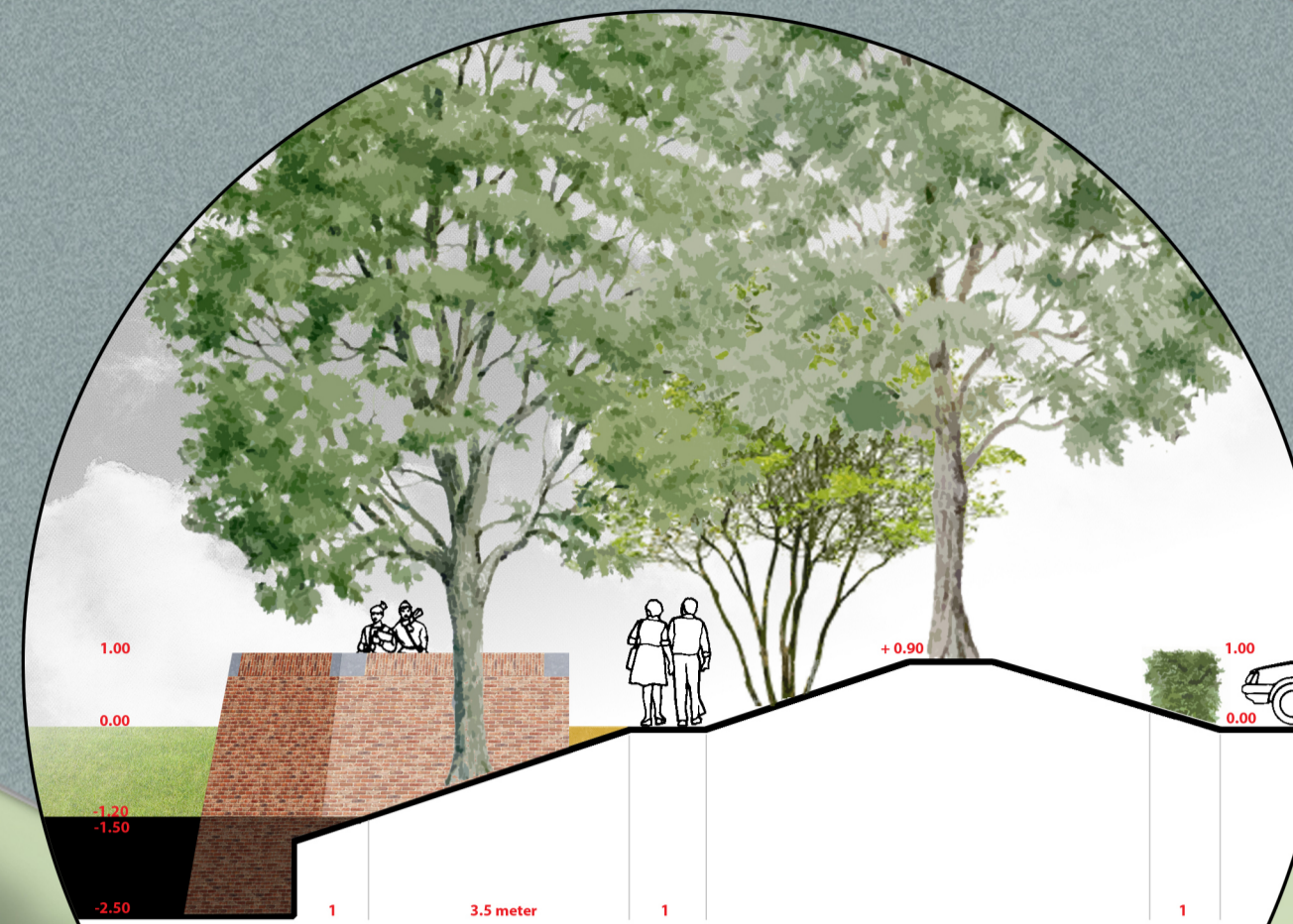
doorsnede: vijver, bastion, pad, heuvel, parkeren
