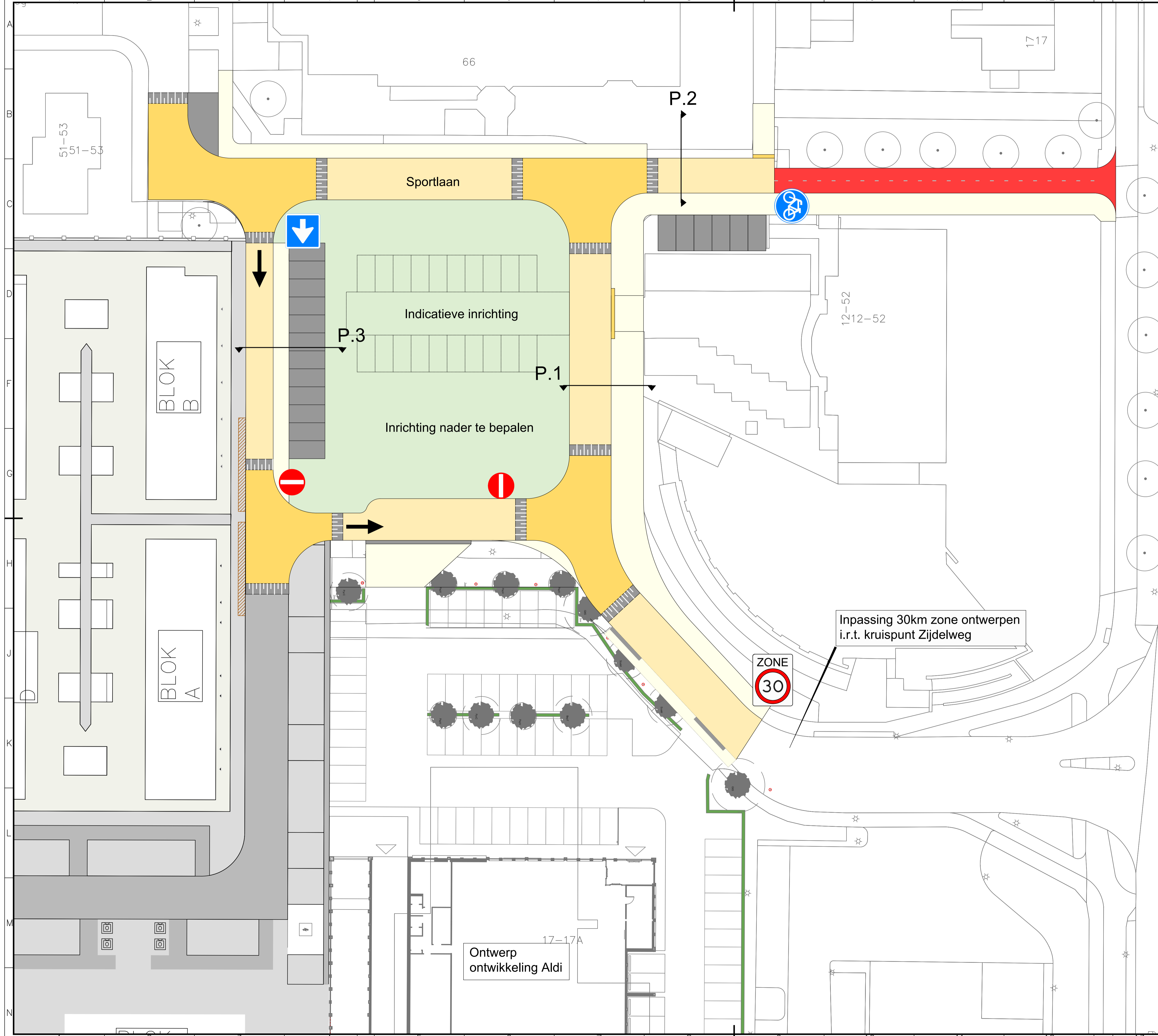
P.1 Verkeersruimte Erftoegangsweg 30 km/uur (gemengd verkeer)
